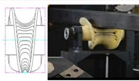
自动上下料装置 多截面管材托架
